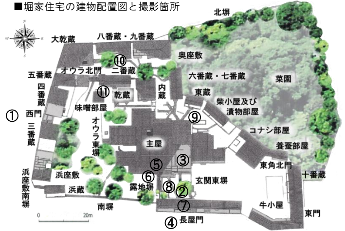
■堀家住宅の建物配置図と撮影箇所
