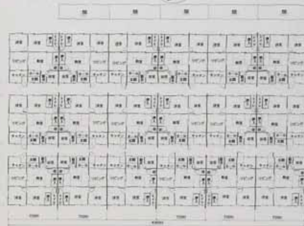
現在 平面図 1:200
