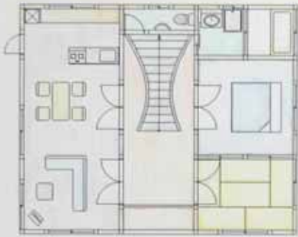
1階平面図 1/200
