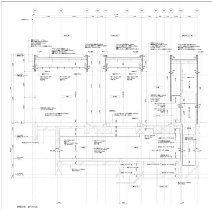
断面詳細図
