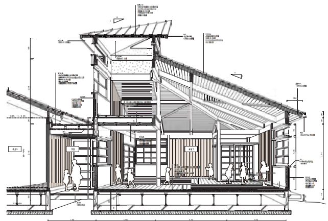
教室7 断面パース
