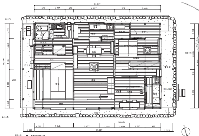
1階平面図
