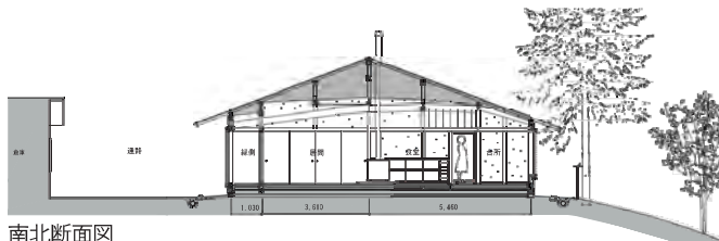
南北断面図
