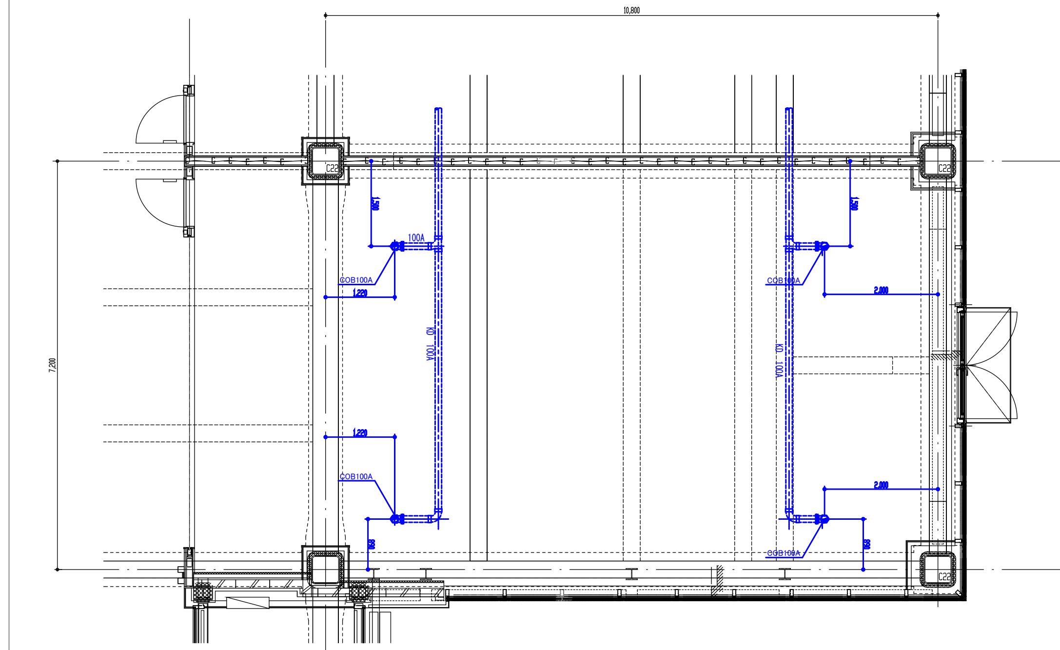
図 5.6-13 排水設備工事図
